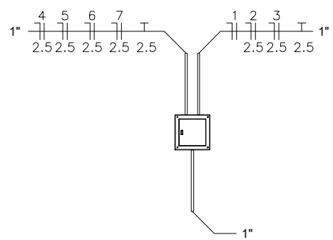
Detalhe do quadro de energia - Quadra
