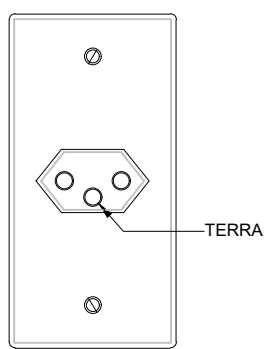
Detalhe tomada 2P+T
