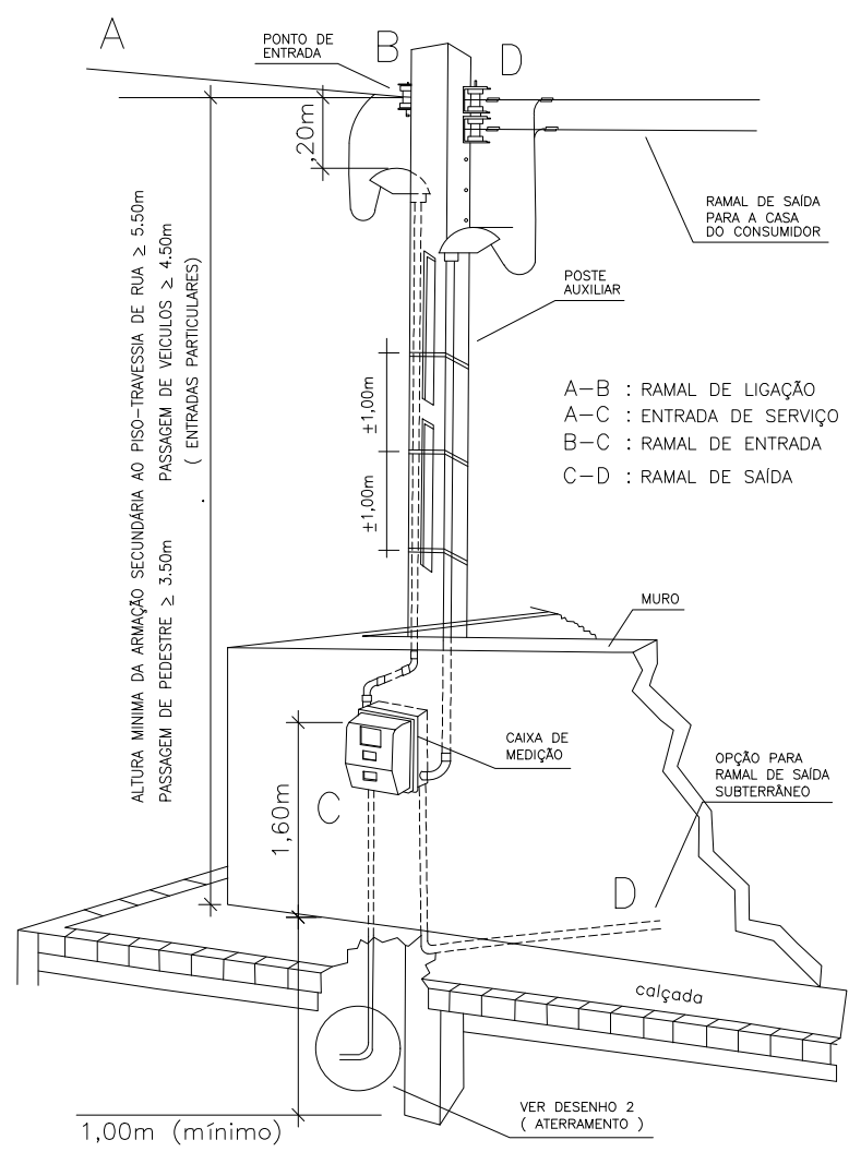
Detalhe de entrada de energia
