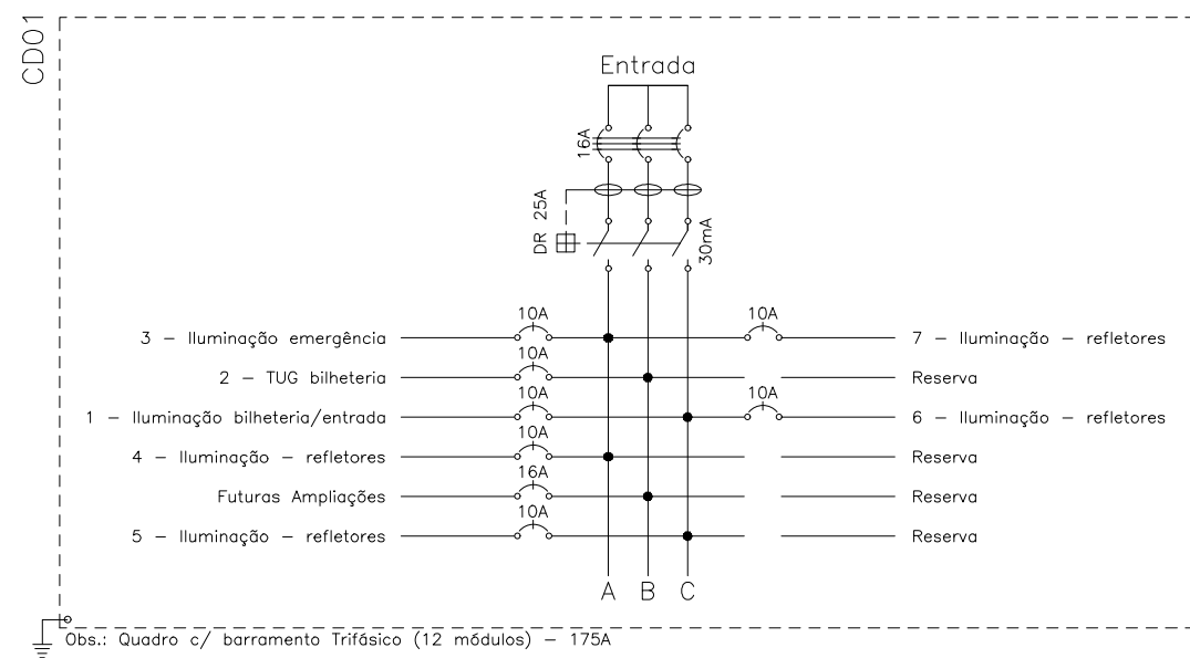
Diagrama Unifilar - Quadra
